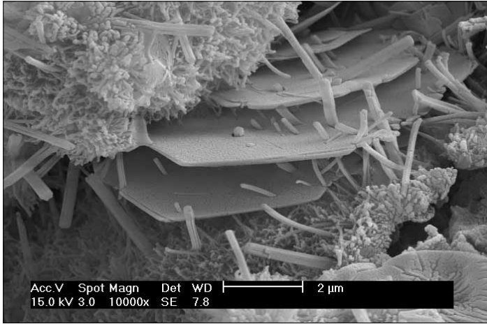
Hidratación del aglomerante a base de cemento Portland de un rejuntdo normal
